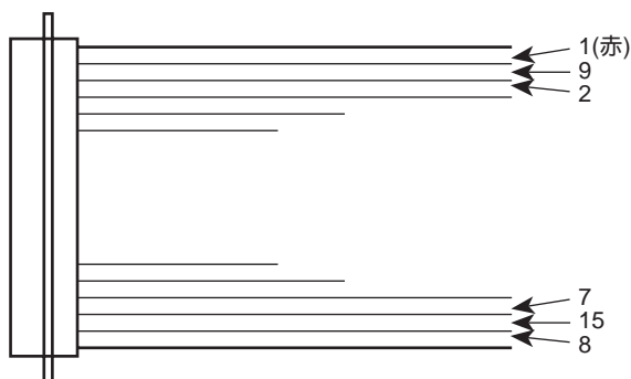
ケーブル 15芯フラットケーブル 導体サイズ：AWG#28
