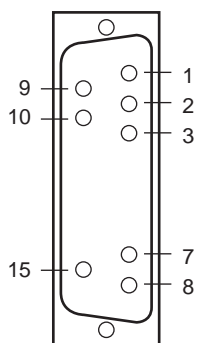
使用コネクタ 15ピンD-Subコネクタ[M(雄)タイプ] スクリューピッチ：インチネジ(#4-40UNC)
